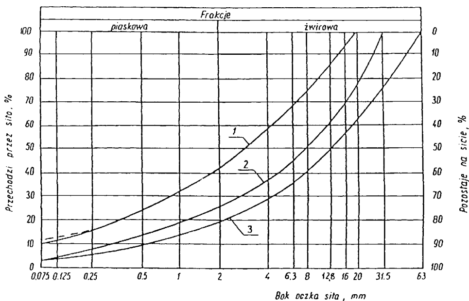
Rysunek 1. Pole dobrego uziarnienia kruszyw przeznaczonych na podbudowy wykonywane metodą stabilizacji mechanicznej 1-2 kruszywo na podbudowę zasadniczą podbudowę jednowarstwową
