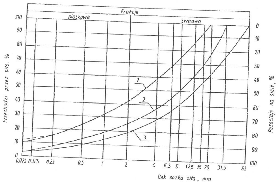
Rysunek 1. Pole dobrego uziarnienia kruszyw przeznaczonych na podbudowy wykonywane metodą stabilizacji mechanicznej 1-2 kruszywo na podbudowę zasadniczą podbudowę jednowarstwową
